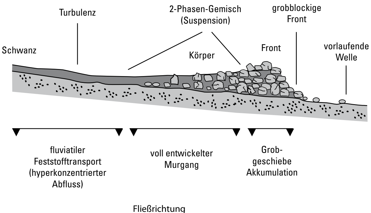
Abbildung 14: Längsschnitt durch einen Murschwanz (modifiziert nach Pierson, 1986)
